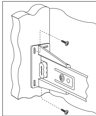
FR 5000 Soporte montaje trasero #2
