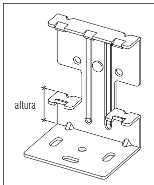
FR 5000 Soporte montaje inferior para marco frontal con offset
