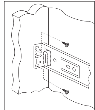
FR 5000 Soporte montaje trasero #2
