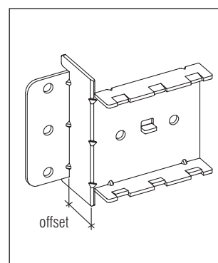
FR 5043 Soporte montaje frontal para marco frontal con offset #2
