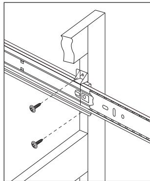
FR 5000 Soporte montaje frontal para marco frontal #2
