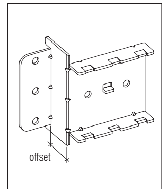
FR 5000 Soporte montaje inferior para marco frontal con offset
